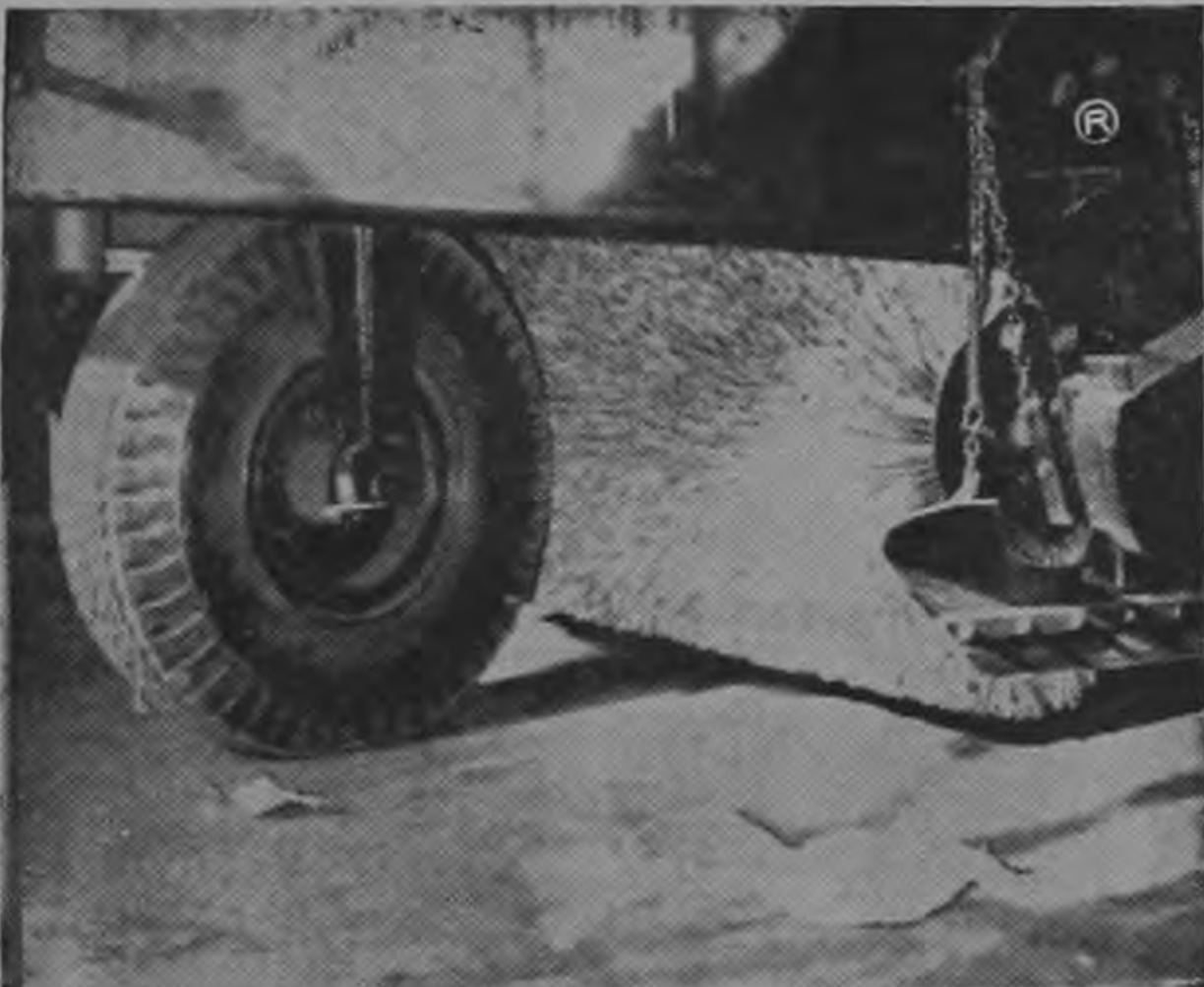
Sección interior de la barredora, donde puede observarse un cepillo cilíndrico que al barrer empuja los residuos hasta una cinta que luego los lleva a un tanque de almacenamiento.
